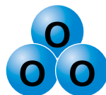
オゾン ( O_3 )
