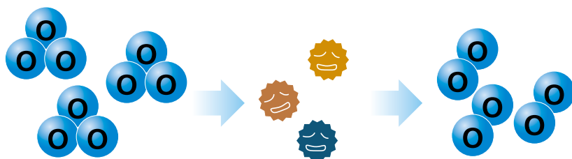
オゾン ( O_3 )
